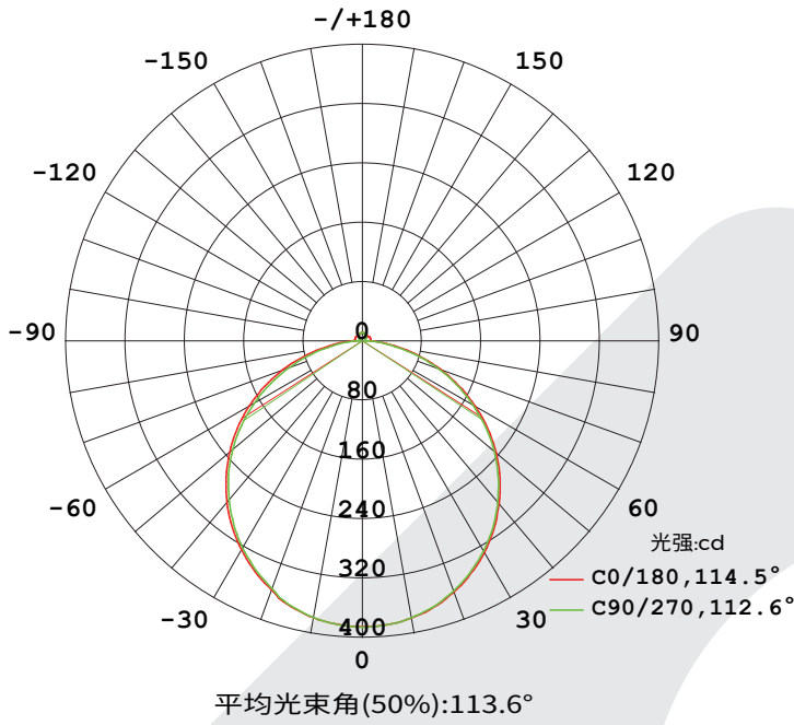
配光曲线
